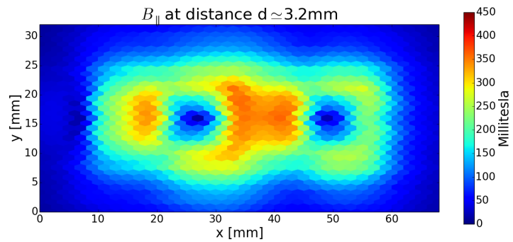
(d) Measurement at 3.2 mm above the unit
